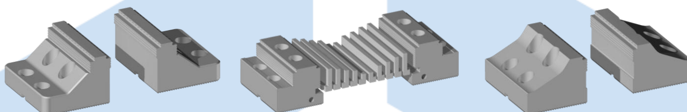
Ganasce di presa alte
