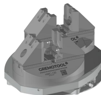
Mors: 2x 837703-B120 Dispositif de serrage: 2x HMC-120
