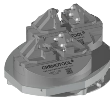
Mors: 2x 837703-B120 Dispositif de serrage: 2x HMC-120
