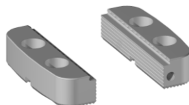
Mors standard SC-LC à griffes
