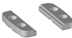
Stufenbacke Niedrig Nr. 837410-BXX
