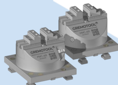
PMC-60I / HMC-60I auf Grundplatte
